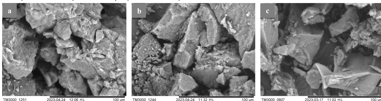
Figure 5. SEM images a) D5-G1-I, b) D9-G2-I, c) D13-G3-I.
